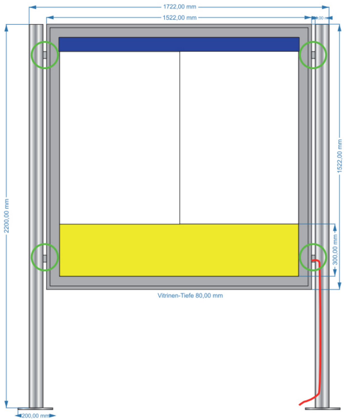
Joonis 2. Reklaamtahvli tehniline lahendus. Hoone fassaadile paigaldatase tugipostide vaheline osa.
